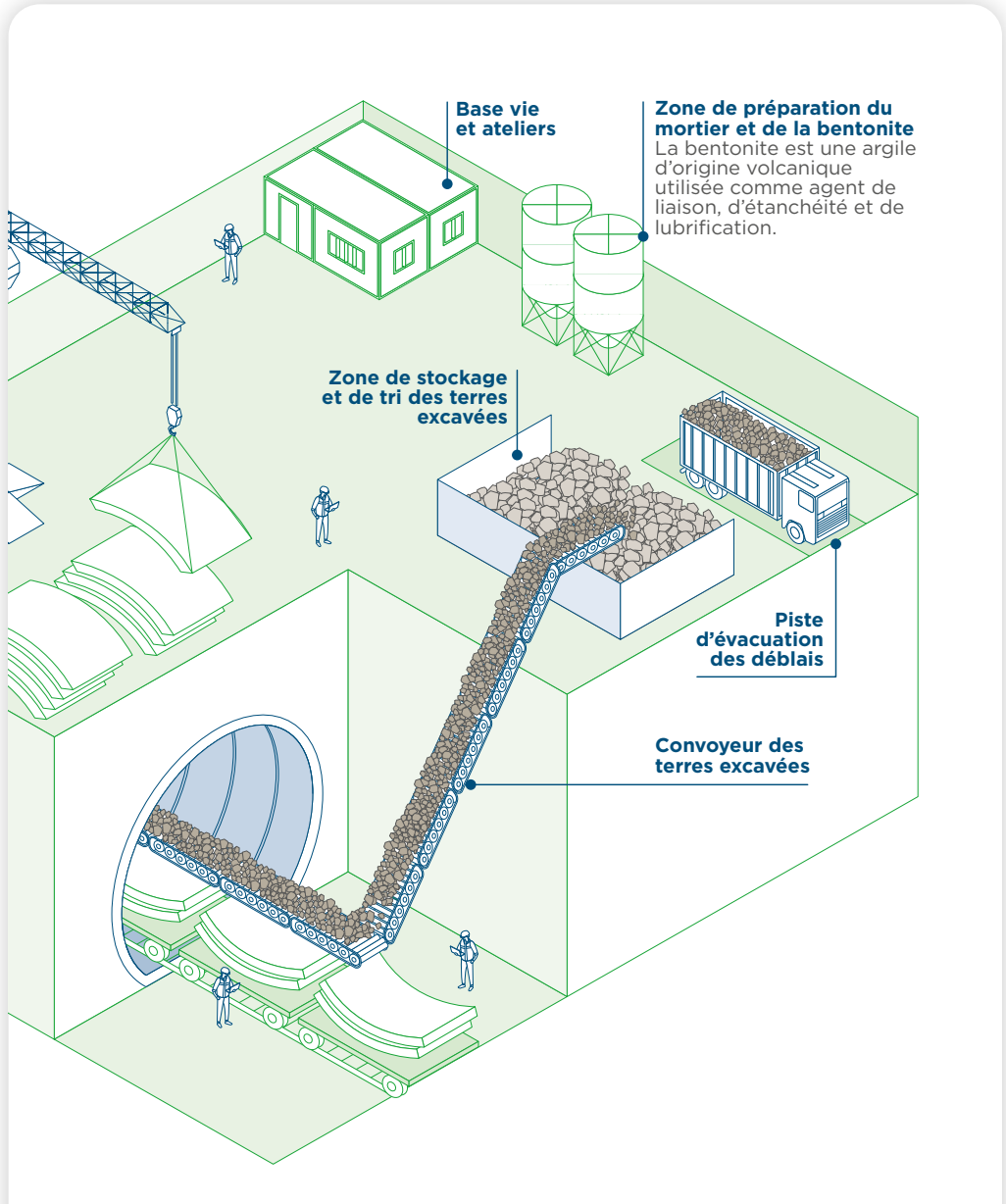
Création d'un schéma d'emprise chantier tunnelier
